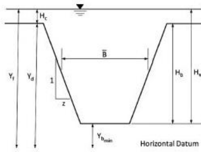
Şekil 2. Froehlich (2008) modelinde kullanılan idealize yamuk yarık kesiti.
