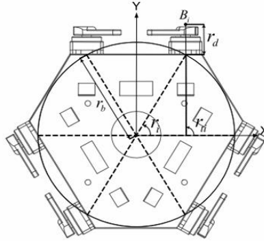
Şekil 2. Bivektörü ve açılarının gösterimi
