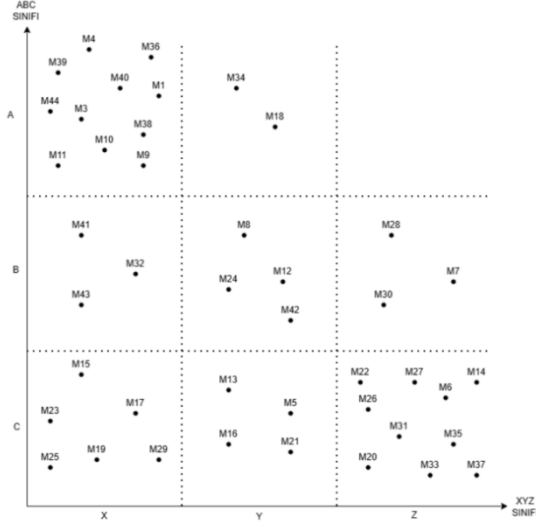
Şekil 1. 44 ürünün 2024 yılı ABC-XYZ Grafiği
